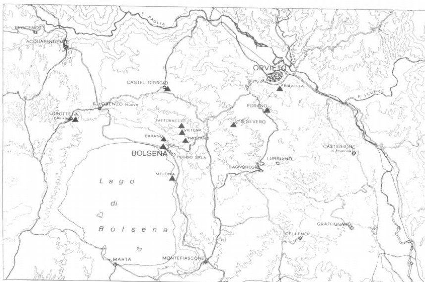
Fig. 1. — Diffusion des inscriptions súōna dans le territoire de Volsinies. (d'après les provenances signalées dans le CIE, III, 2 et les ETT)
